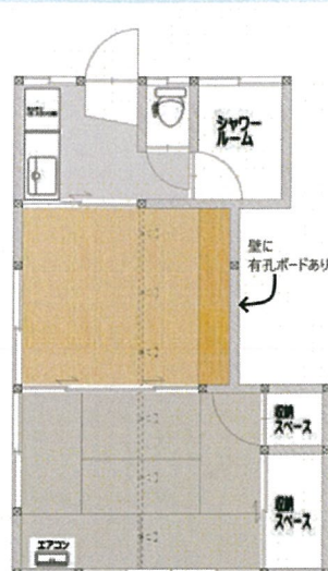
間取り図(平面図)
